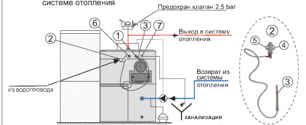
Схема 2. Монтаж термической защиты котла ECO-CK Plus 25/35 при закрытой системе отопления
