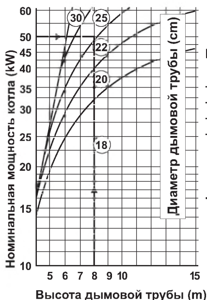
Рис 4. Размеры дымовой трубы для котла ECO-CK Plus
