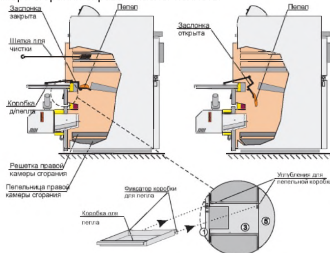
Рис 9. - Камера сгорания справа - масло/ пеллеты
