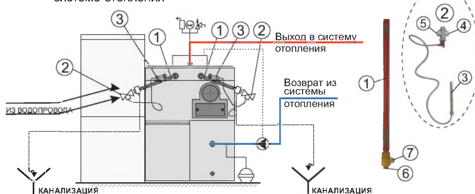
Схема 2.1. Монтаж термической защиты котла ECO-CK Plus 50 при закрытой системе отопления
