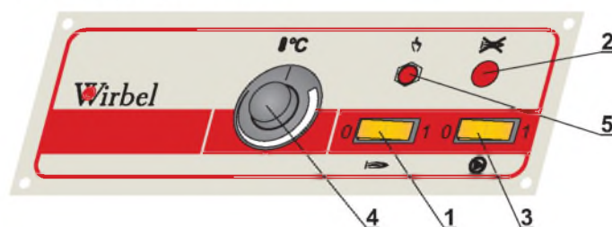
Рис 5. Основная регулировка котла
