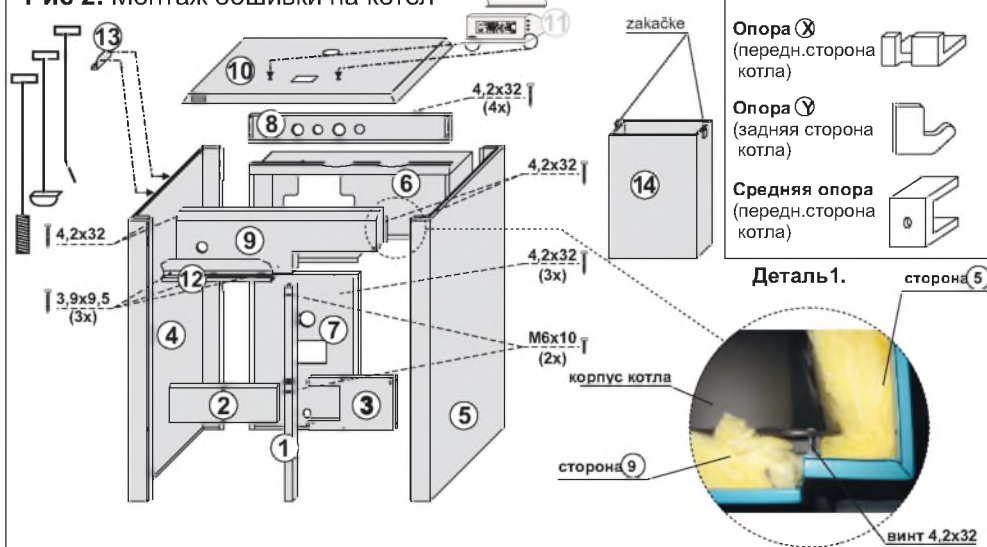
Рис 2. Монтаж обшивки на котел
