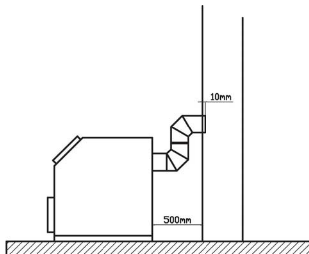
Неправильное подключение
