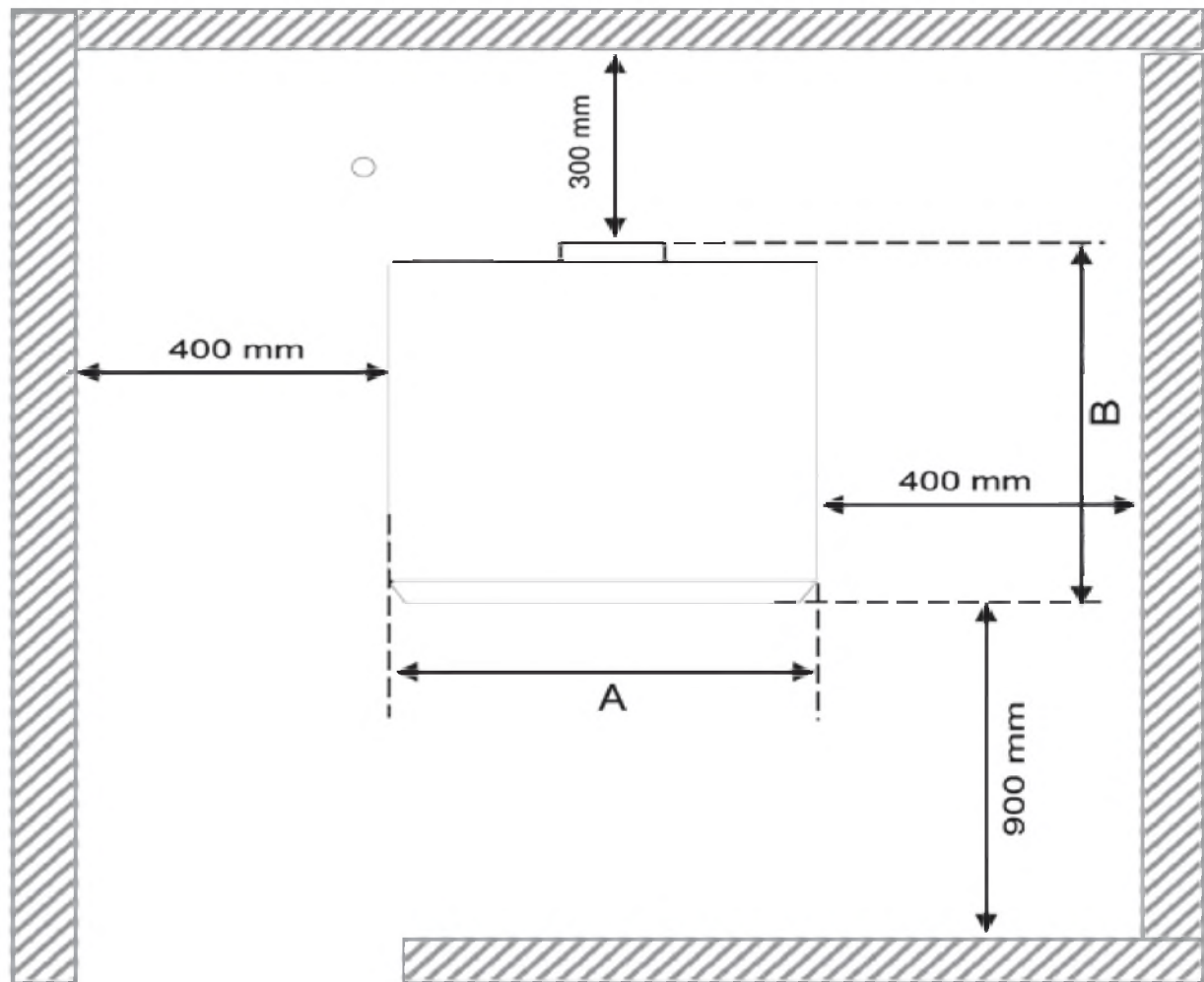
Рис. 3. Установочные размеры.
