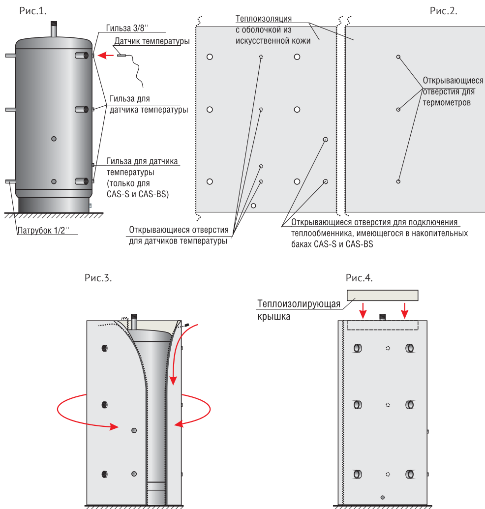
Рис.1-7. Порядок монтажа теплоизоляции на бак-аккумулятор тепла
