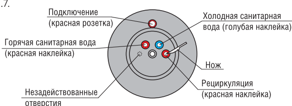
крышка для CAS-B и CAS-BS
