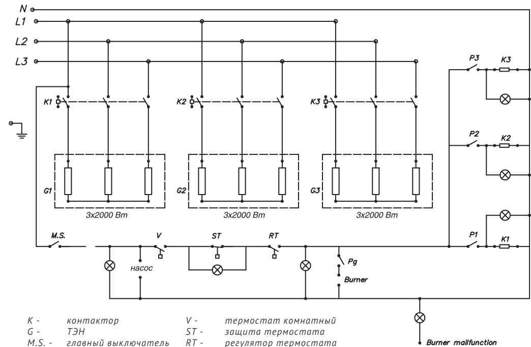
Рис.12. Схема электрических подключений ТЭНа 18 кВт
