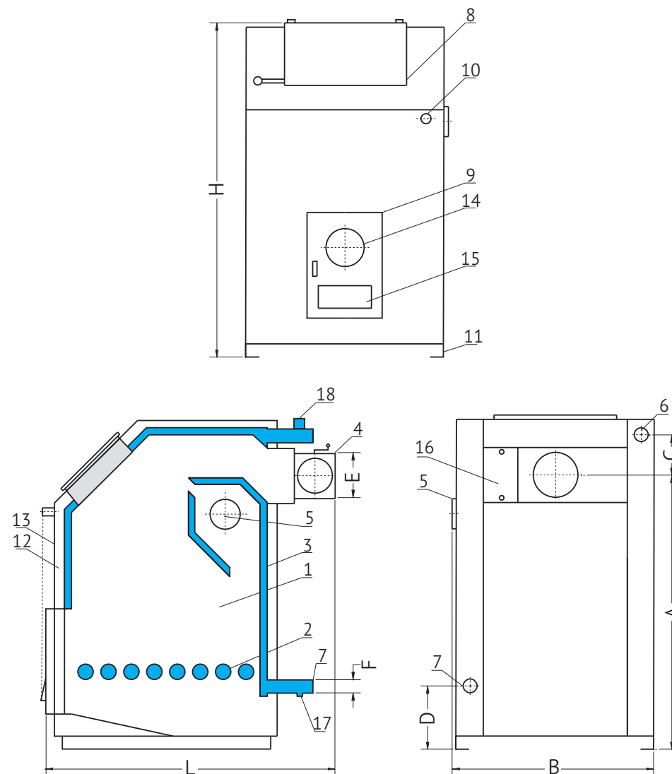
Рис.1. Вид котла ЕКО
